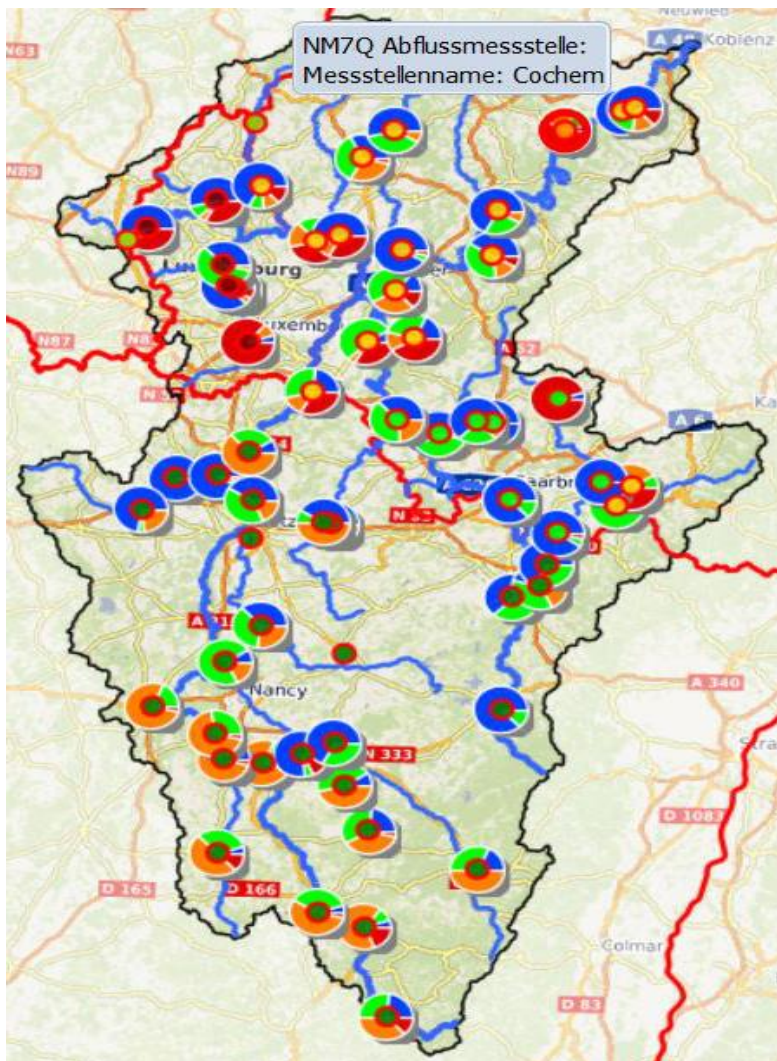
Karte 2: Übersichtskarte des jährlichen Niedrigwassermonitorings. (5-farbige Legende: siehe oben unter "Festlegung gemeinsamer Abflussschwellenwerte und Klassifizierung der Intensität von Niedrigwasser")
